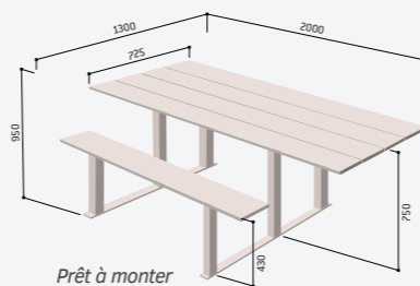
Prêt à monter
