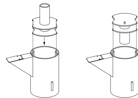
Position d'accueil borne
